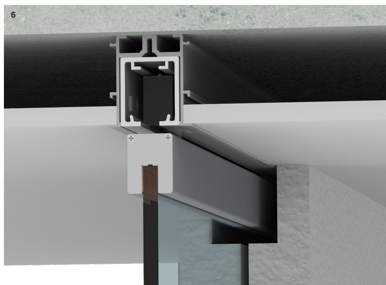
1, 2 y 3 Conjunto perfil Fundas FT XL + Perfil Star XL, montaje a falso techo I Support FT XL + Star XL track set, false ceiling mounting I Ensemble Rail de couverture FT XL + Star XL, fixation a faux-plafond. 4, 5 y 6 Conjunto perfil Fundas FT XL + Perfil Star XL, montaje entre paredes I Support FT XL + Star XL track set, mounting between walls I Ensemble Rail de couverture FT XL + Star XL, fixation entre les murs.
