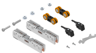
2 x1 Juego de accesorios | Fitting set | Garniture SV-P70 EASY x2 Freno retenedor | Retaining stopper | Frein de retenue
