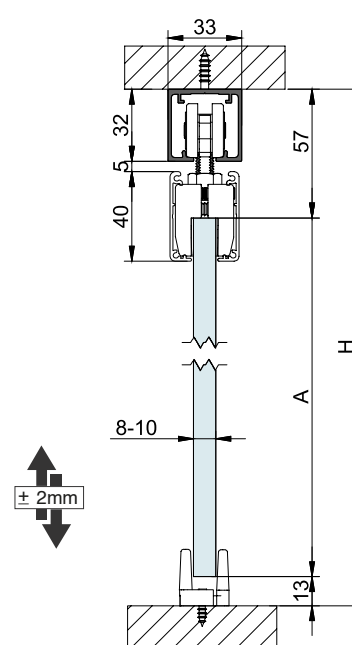
STAR A= H-70
