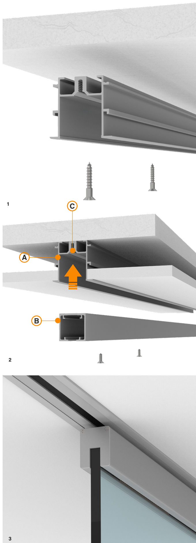
A Perfil funda FT | Support FT track | Rail de couverture FT. B Perfil Star | Star track | Rail Star. C Diseño de perfil con avellanado integrado | Track design with drilled countersink | Conception de rail avec fraisage intégré.
